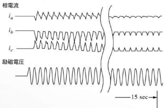
変圧器課電時の励磁突入電流波形
