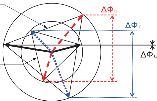
逆位相制御投入〔参考〕 （励磁突入電流が最大級になるケース）
