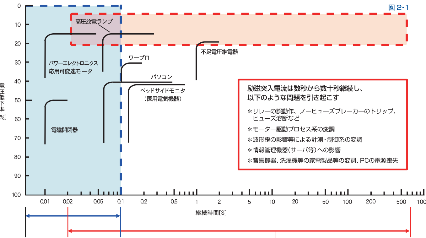
雷撃等の事故遮断による瞬時電圧低下の範囲
