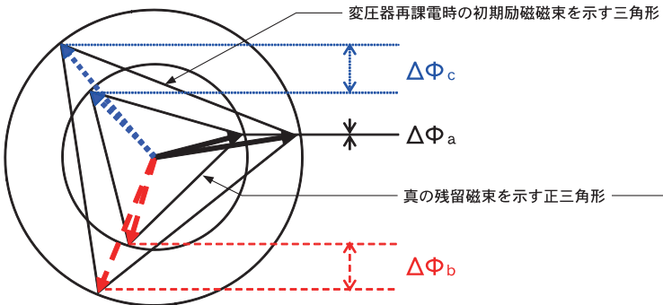
同一位相角投入制御〔本装置で採用〕 （残留磁束最小相スカラー値一致制御）
